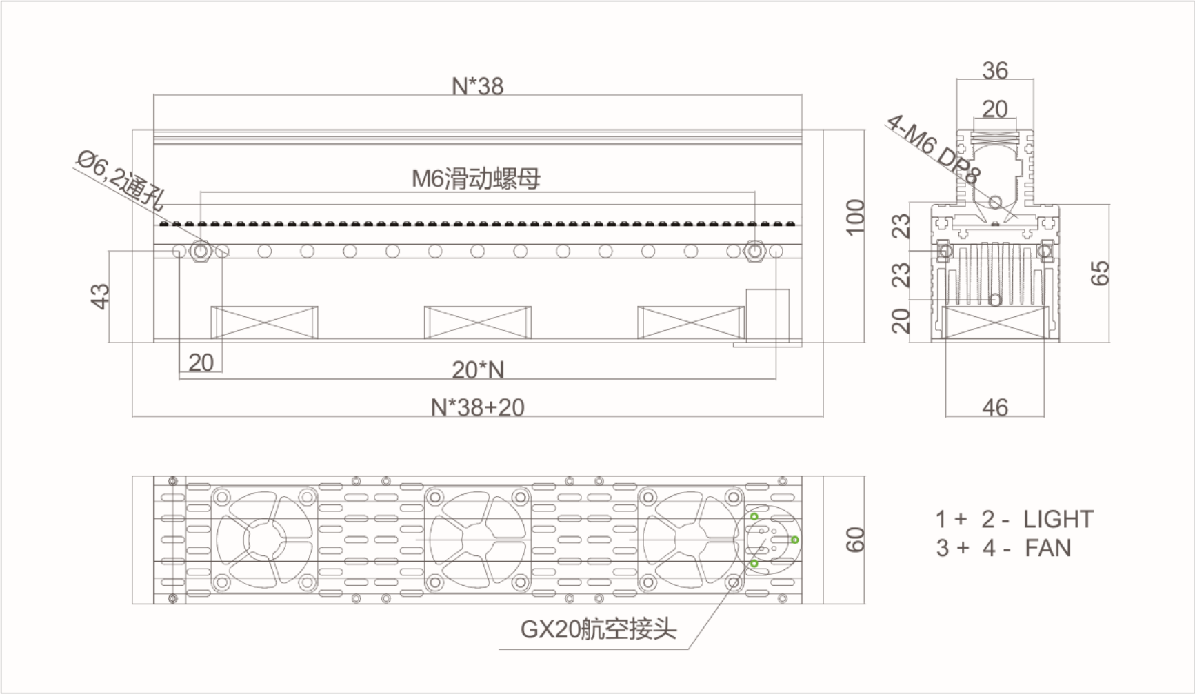
高亮线光源尺寸图
