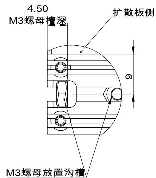
局部视图 B 比例 2 : 1
