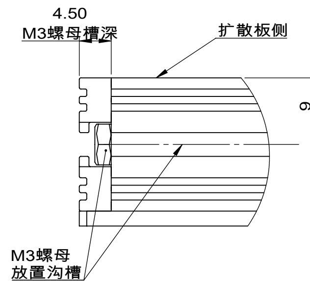
局部视图 B 比例 2 : 1
